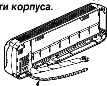
Дренажный шланг
