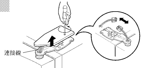
上鉸鏈
