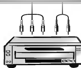
< Pannello posteriore del lettore di DVD >
