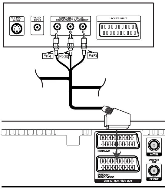
Hátlapja DVD/ videomagnó kombi vevőkészülék
