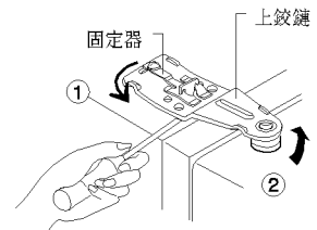
上鉸鏈
