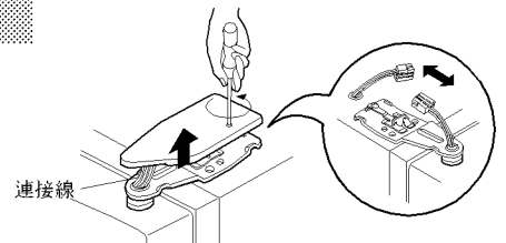
上鉸鏈
