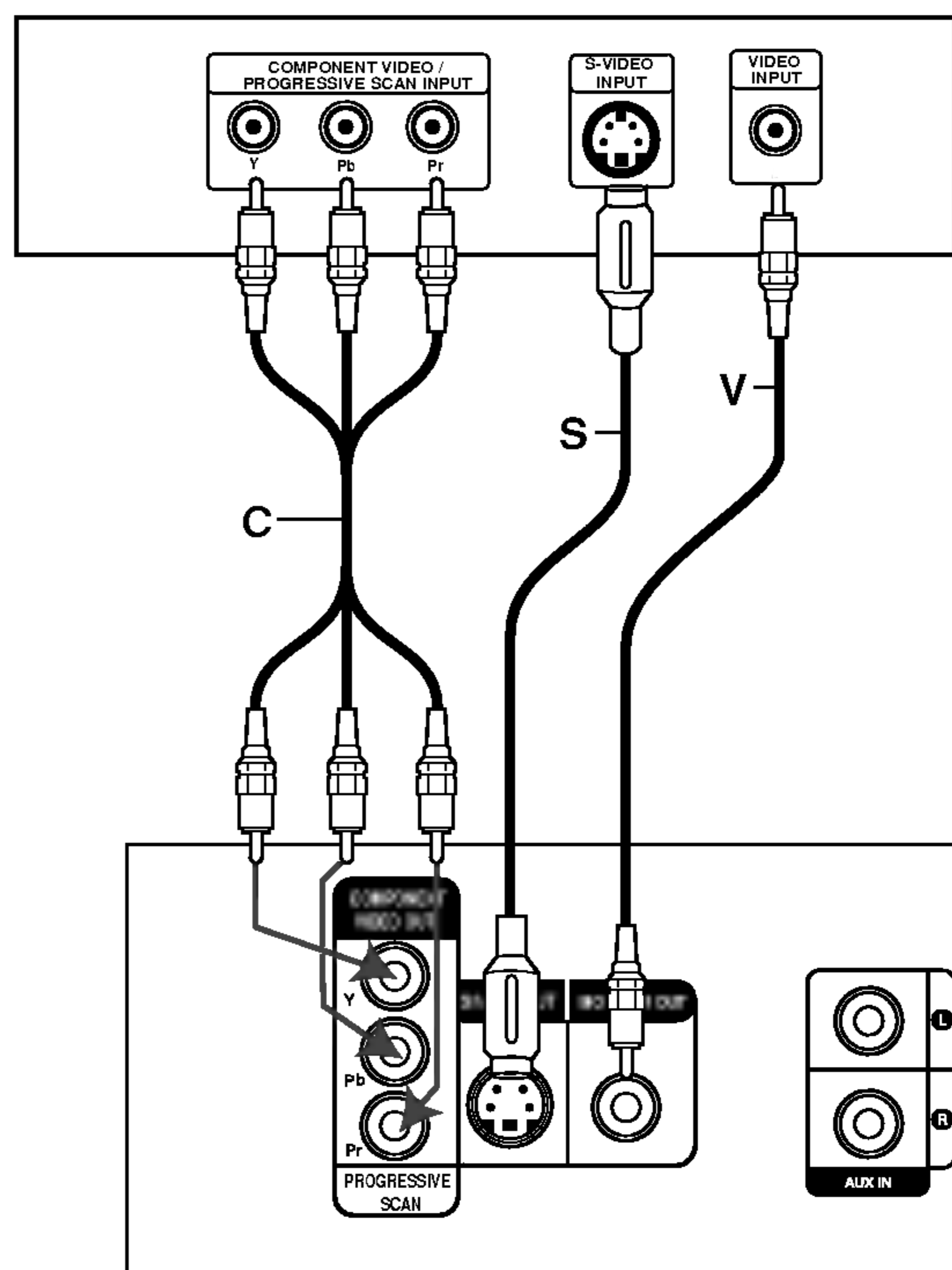
DVD/CD 播放機的背板
