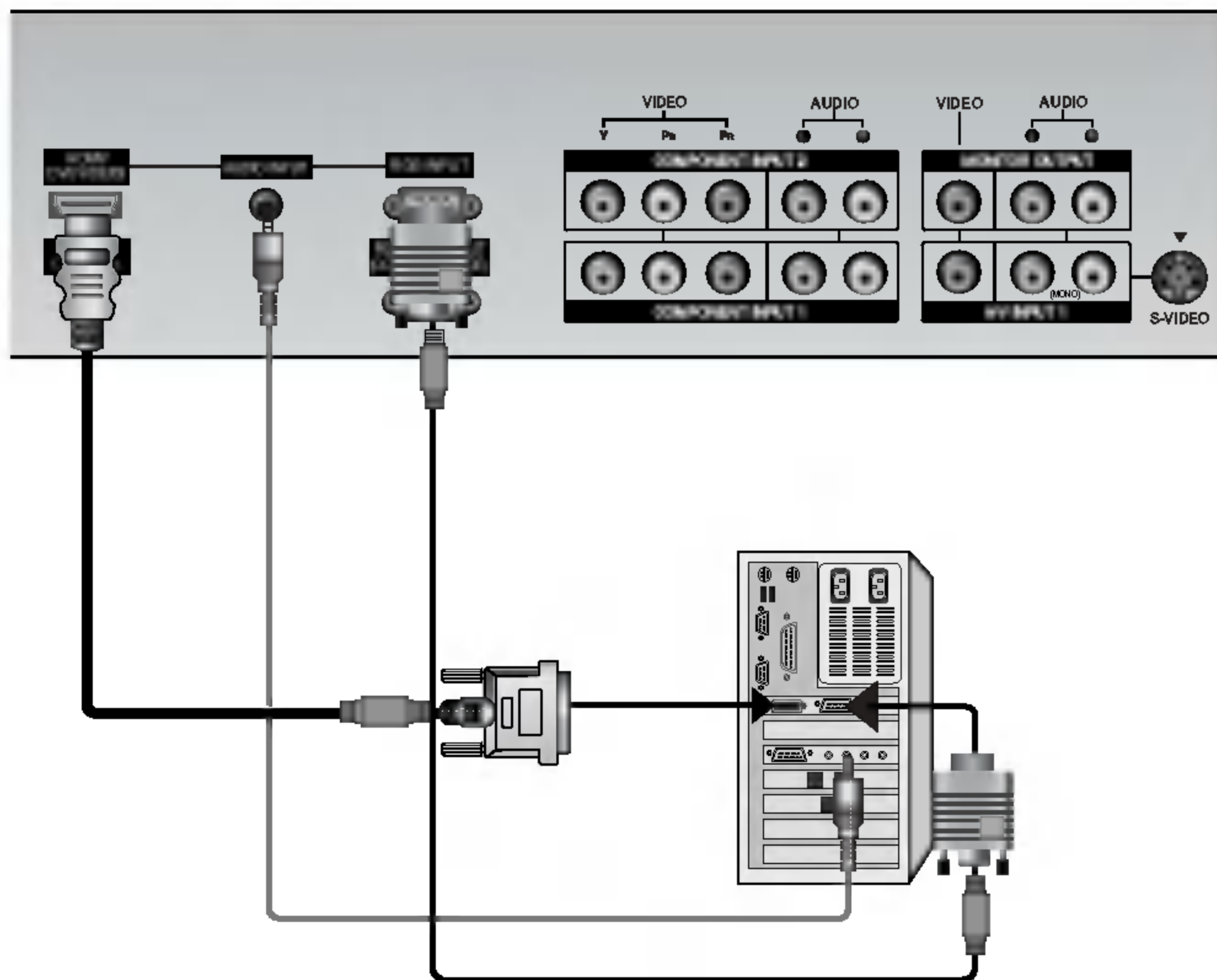
< 电视机后端控制面板 >
