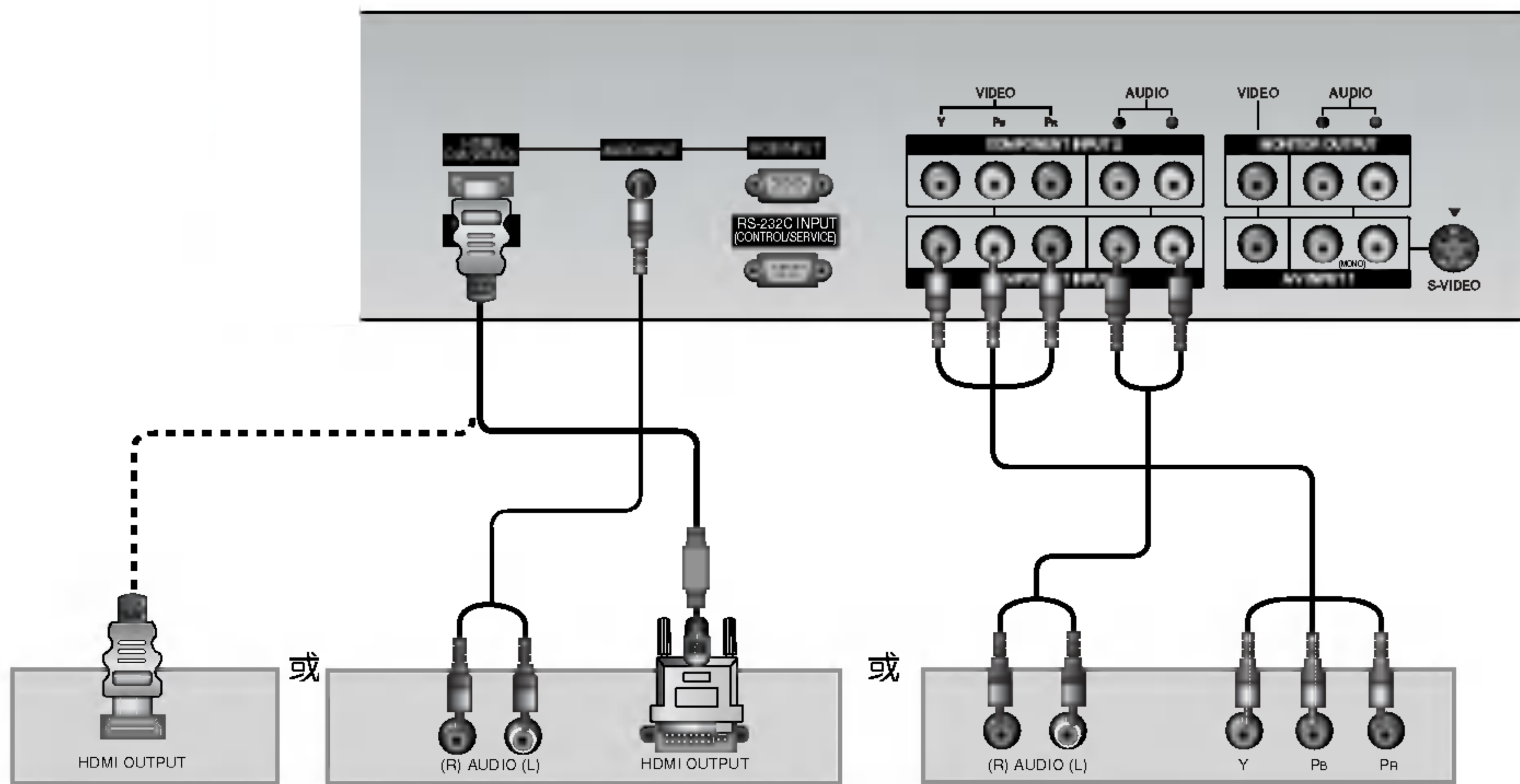
< 数字机顶盒 >
