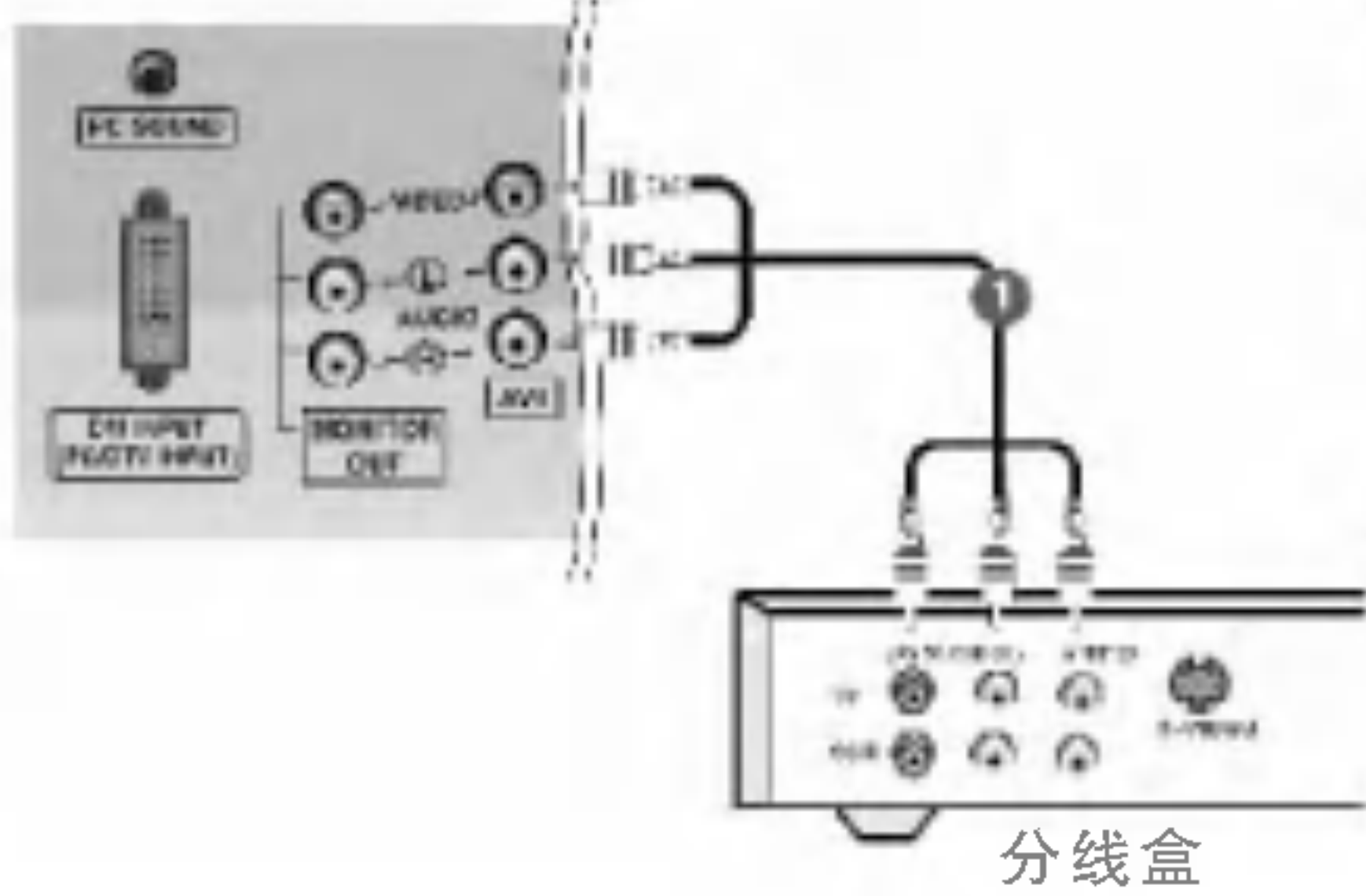
TV后面板
