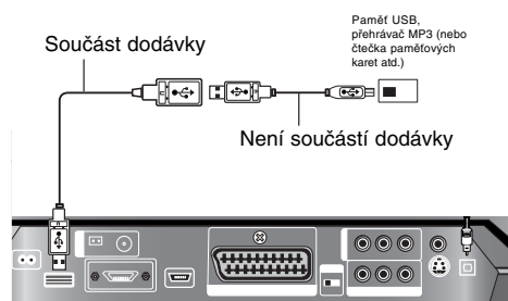
Zadní strana DVD/CD přijímače
