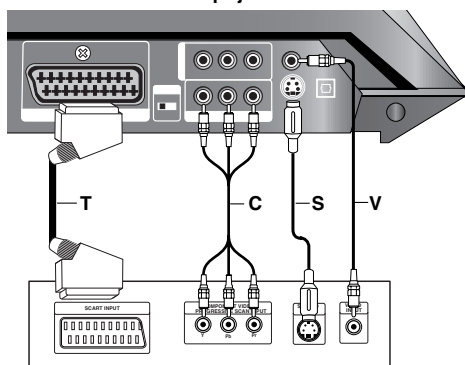
Zadní část televizoru
