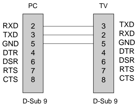
3股线的配置 (非标准连接线)
