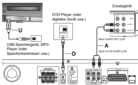
Rückseite des DVD/CD-Receiver
