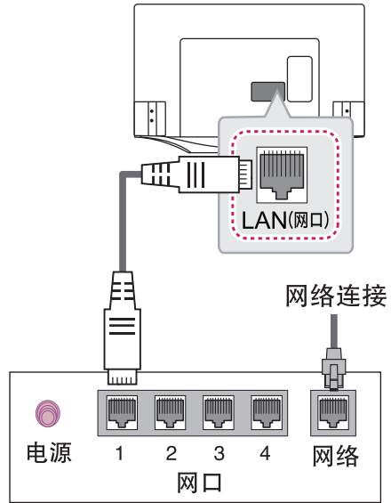
有线路由器
