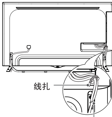
缆线固定器
