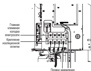
Подсоединение главного провода питания
