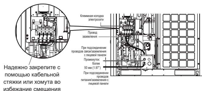
Подсоединение провода связи/заземления
