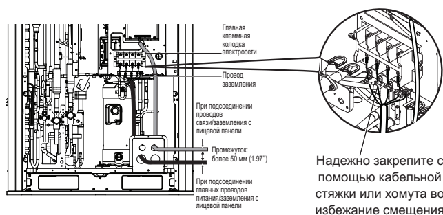
Подсоединение провода связи/заземления
