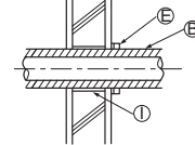
Шахта для трубы на крыше
