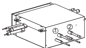
PRHR022 или PRHR022A (2 ответвления)
