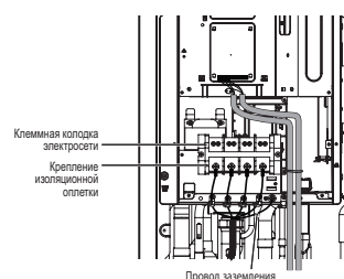
Подсоединение главного провода питания
