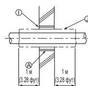
Шахта для трубы на крыше
