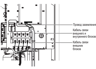
Подсоединение провода связи/заземления
