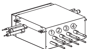
PRHR042 или PRHR042A (4 ответвления)
