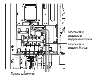
Подсоединение провода связи/заземления
