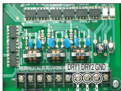
< Hlavná doska plošných spojov vonkajšej jednotky >
