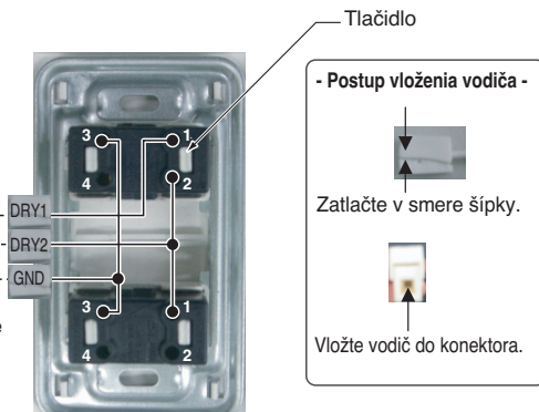
<Zadná strana vonkajšieho suchého kontaktu>
