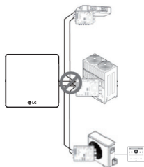
<Λανθασμένο παράδειγμα: RS485 μορφή σύνδεσης αστεριού (STAR)>
