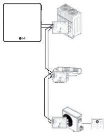
<Σωστό παράδειγμα: RS485 μορφή σύνδεσης δίαυλου (BUS)>
