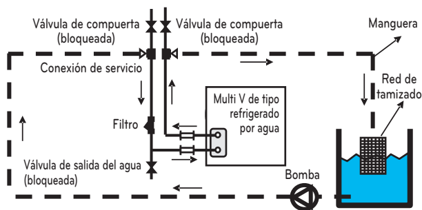
[Limpieza del intercambiador de calor de paneles]
