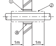
Porci3n entrante en el limite de fuego y pared limite
