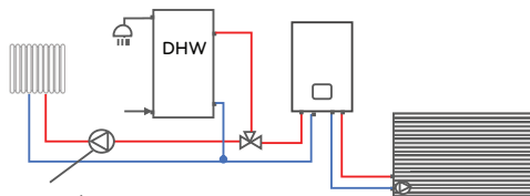
Pompe externe
