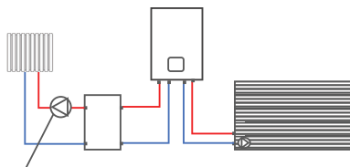
Pompe externe
