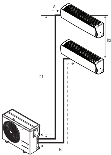
Тип связи труб
