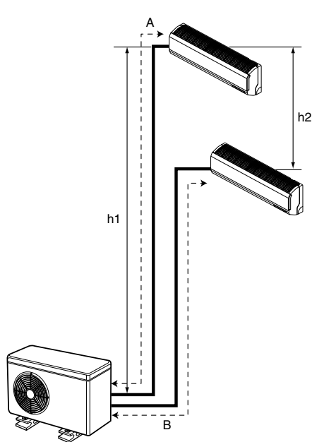
Tipo multitubería
