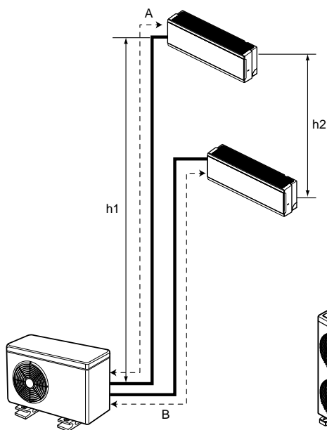
Type tuyauterie multiple
