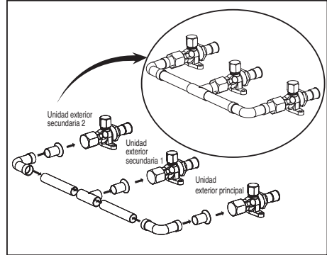
3 unidades exteriores
