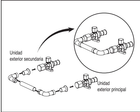
2 unidades exteriores
