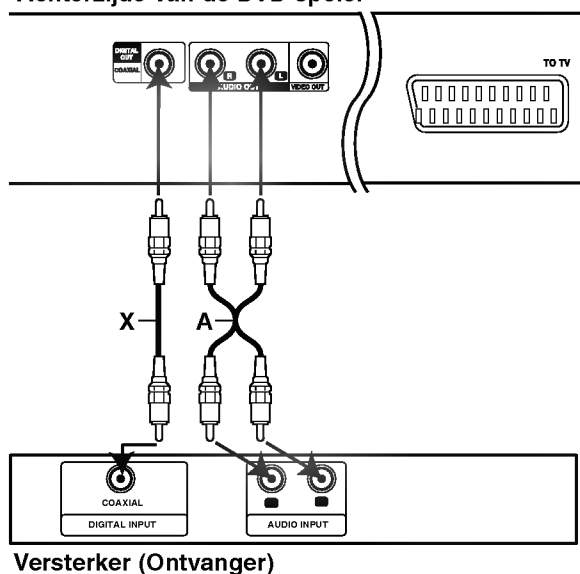
Achterzijde van de DVD-speler
