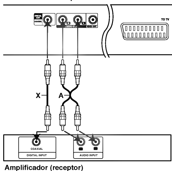
Painel traseiro do aparelho de DVD
