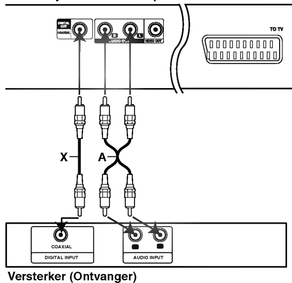
Achterzijde van de DVD-speler
