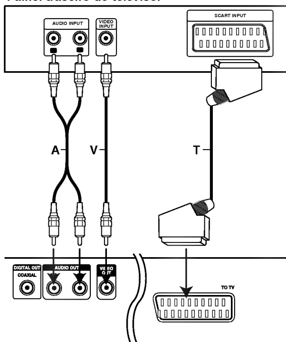
Painel traseiro do aparelho de DVD
