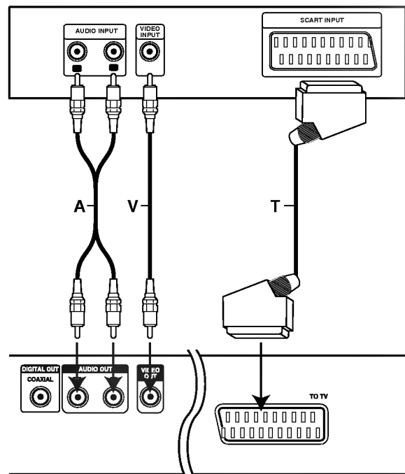
Achterzijde van de DVD-speler
