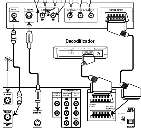
La parte trasera de esta unidad (Conexión básica)
