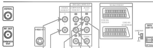
La parte trasera de esta unidad (Conexión de un Vídeo Componente)
