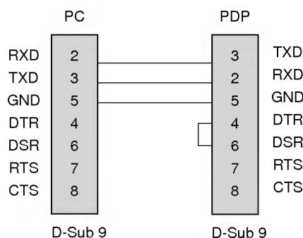
3-johtiminen kaapeli (ei standardi)
