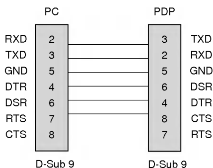
7-johtiminen kaapeli (standardin RS-232C mukainen kaapeli)
