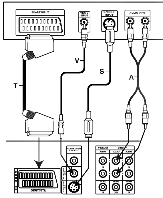
Заден панел на DVD/CD ресивъра
