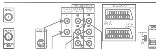
Stražnji dio ovog uređaja (Component video spajanje)
