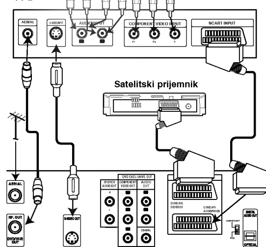
Stražnji dio ovog uređaja (Osnovni priključak)
