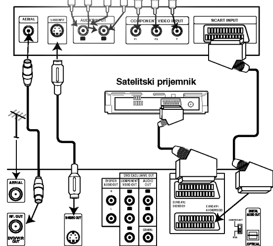
Zadnji panel ovog aparata (osnovni spojevi)
