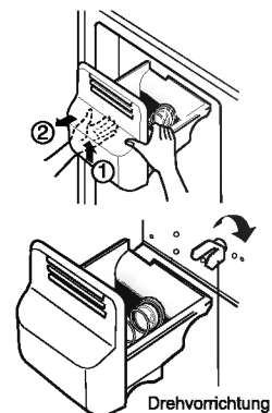
Drehvorrichtung
