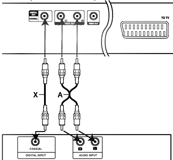
Усилвател (приемник)
