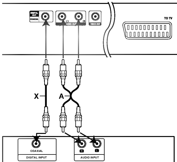
Amplificateur (Récepteur)
