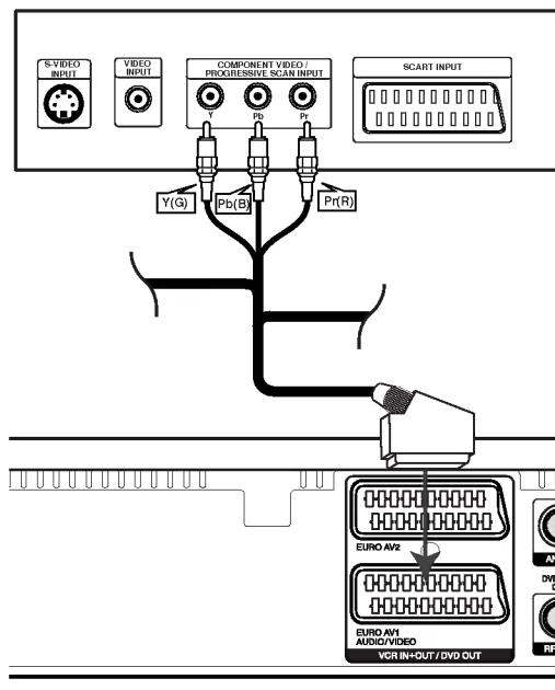
Stražnji panel KOMBINIRANI DVD/VCR
