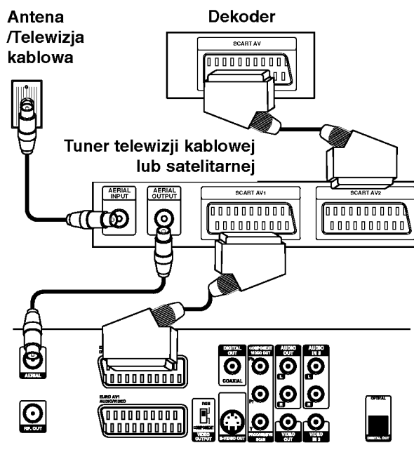
Tył nagrywarki
