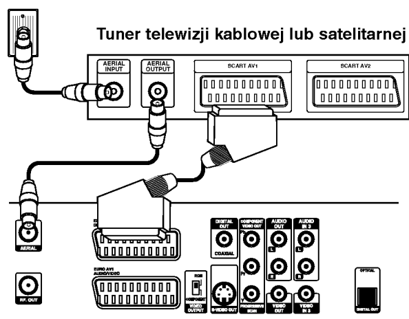
Tył nagrywarki
