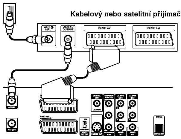
Zadní panel rekordéru DVD
