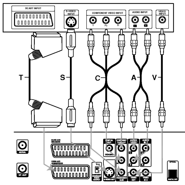
Zadní panel rekordéru DVD
