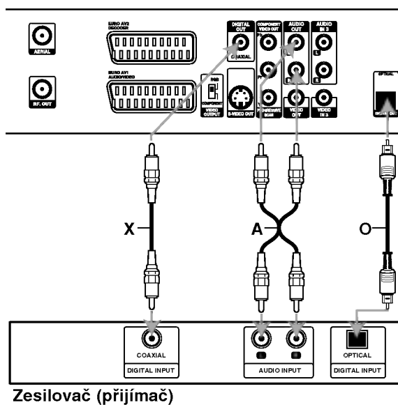
Zadní panel rekordéru DVD
