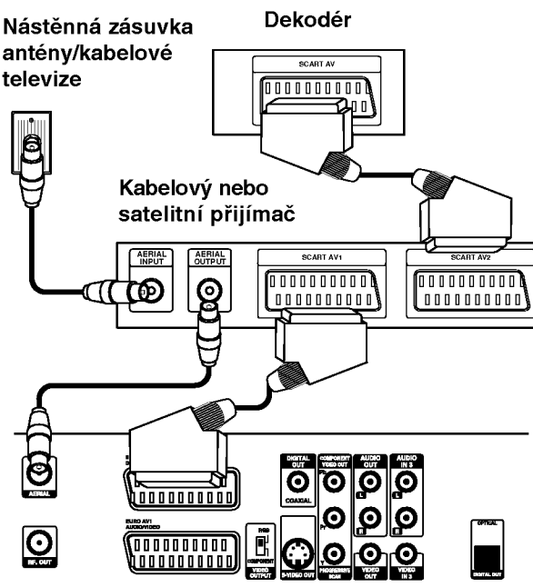
Zadní panel rekordéru DVD
