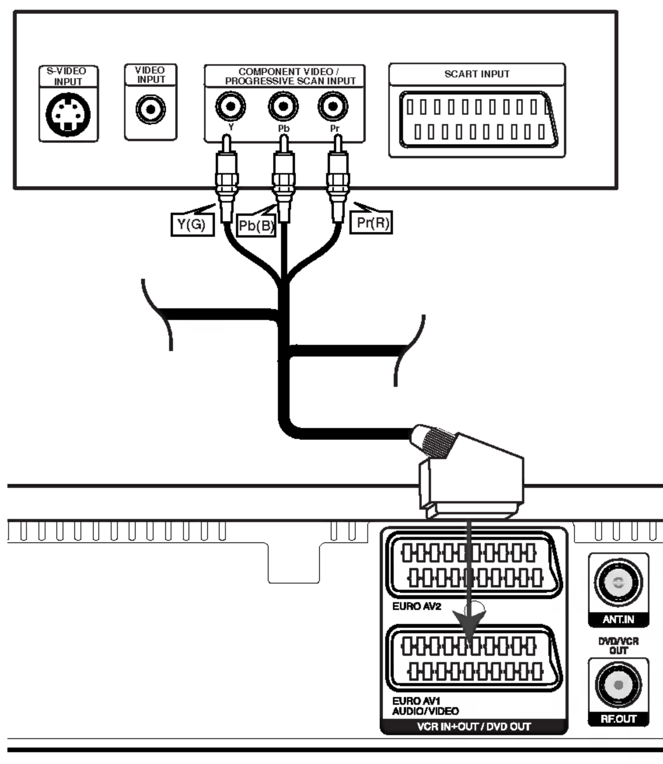
Stražnji panel KOMBINIRANI DVD/VCR
