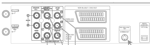
Tył urządzenia (Podłączenie wyłącznie DVD)
