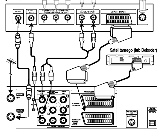
Tył urządzenia (podłączenie podstawowe)
