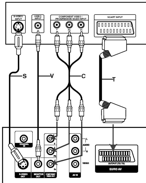
Заден панел на DVD/CD ресивъра
