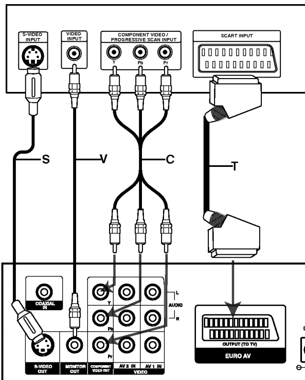
Panneau arrière du récepteur DVD
