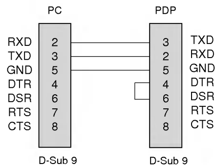
Configuración de 3 hilos (No estándar)
