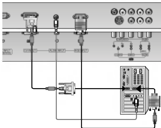
< Achterpaneel van de monitor >
