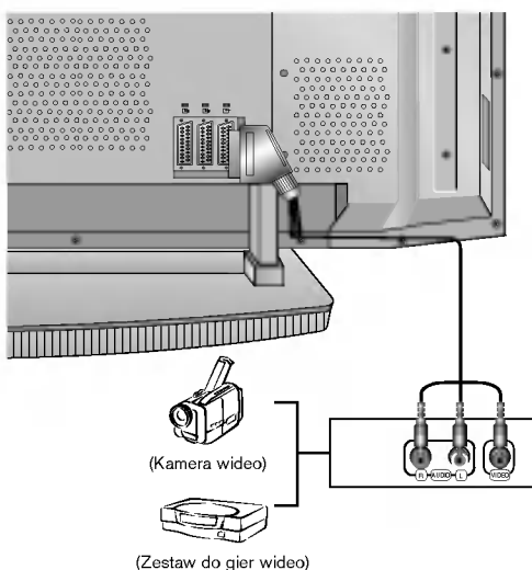
< Tylny panel TV >
