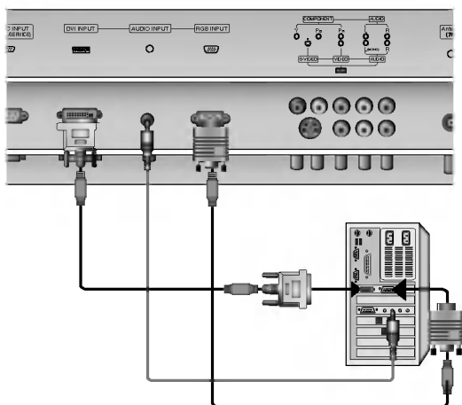
< Tylny panel TV >
