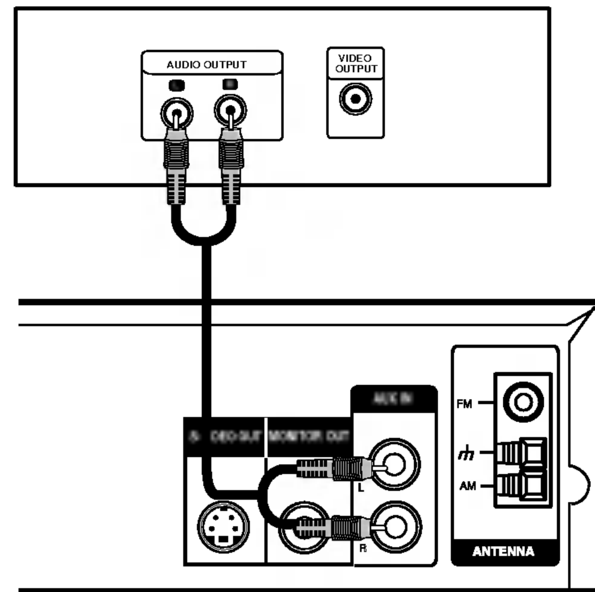
Stražnji dio video rekordera (ili LD playera, itd.)
