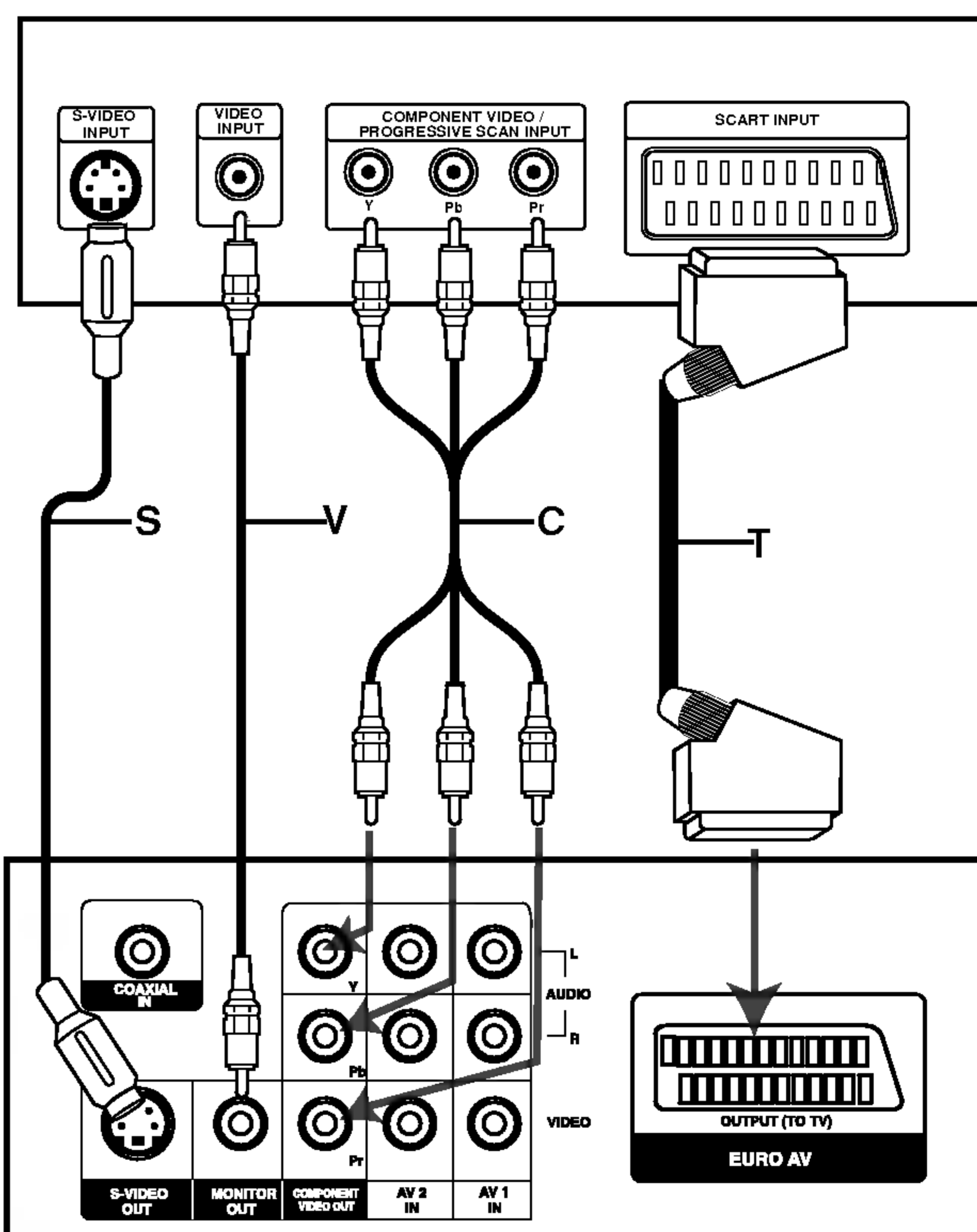
Zadný panel DVD/CD prehrávača
