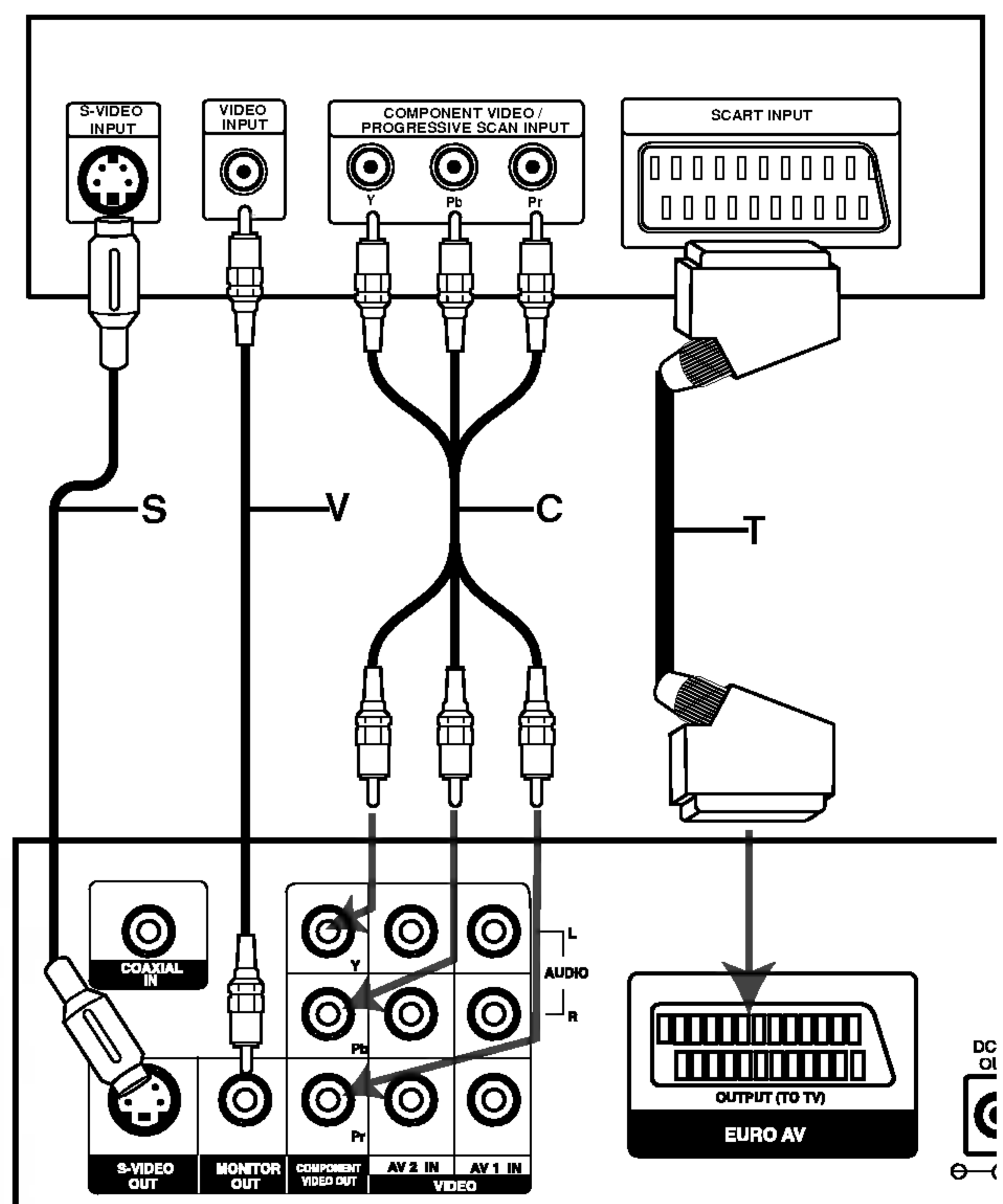
Tylna płyta odbiornika DVD
