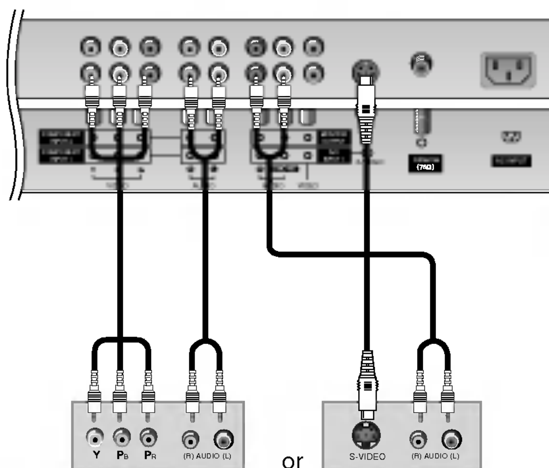
DVD
