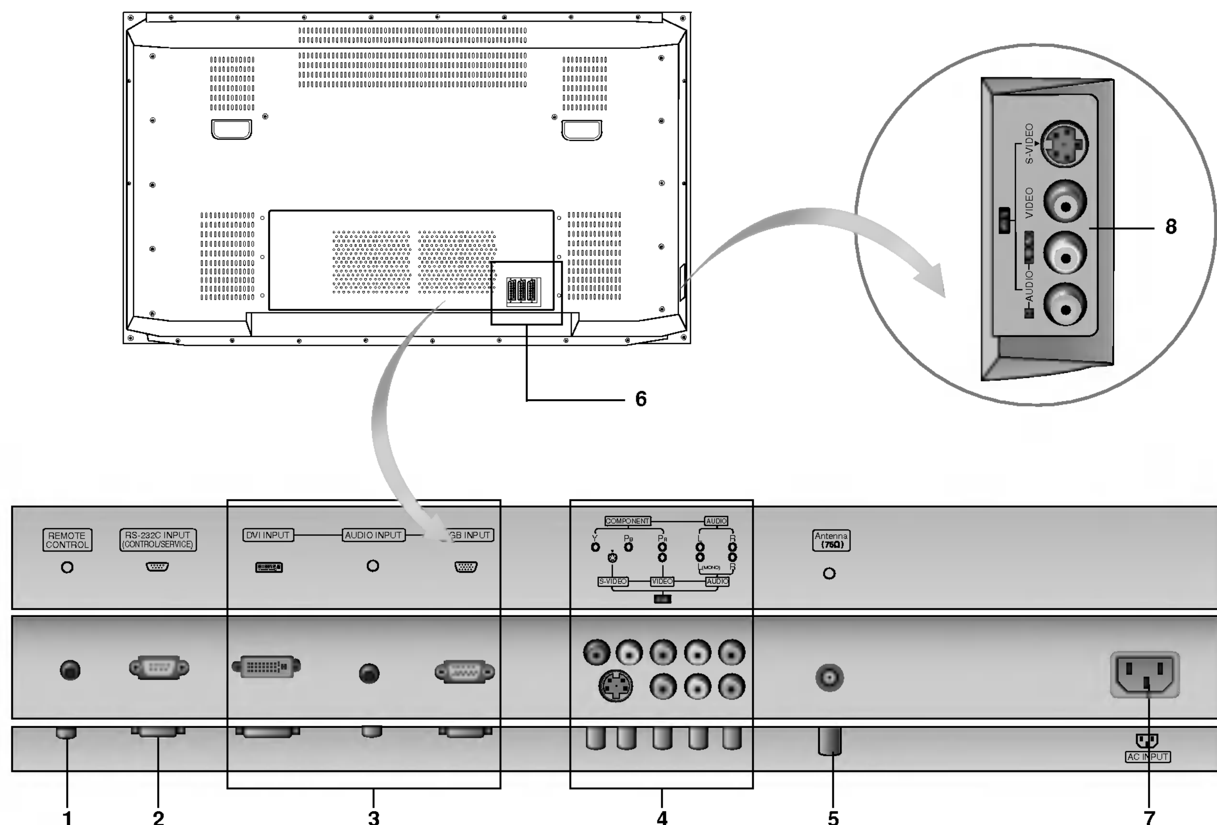
< Panel tylny >
