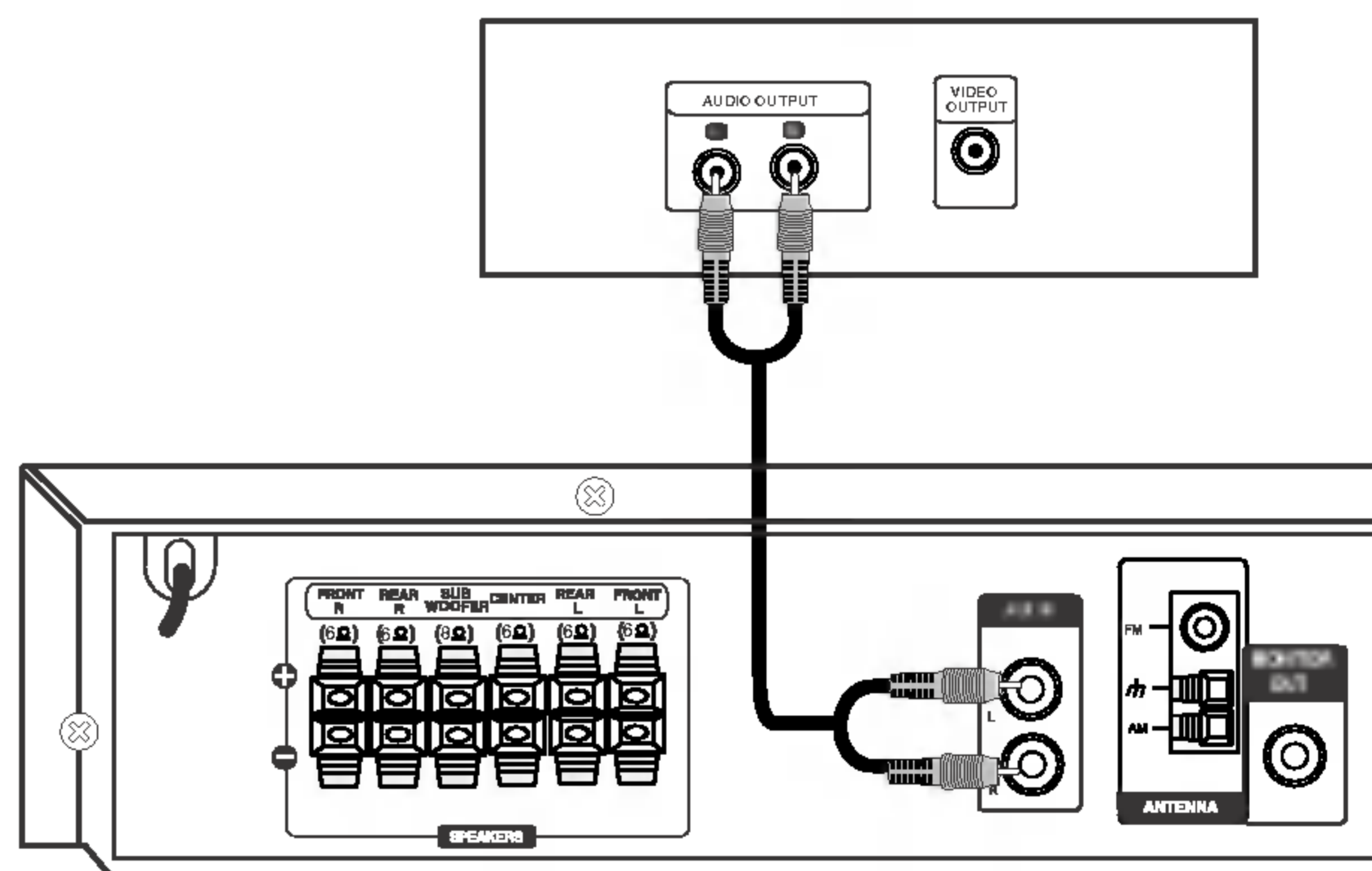
Zadný panel videorekordéra (alebo prehrávača LD, atď.)
