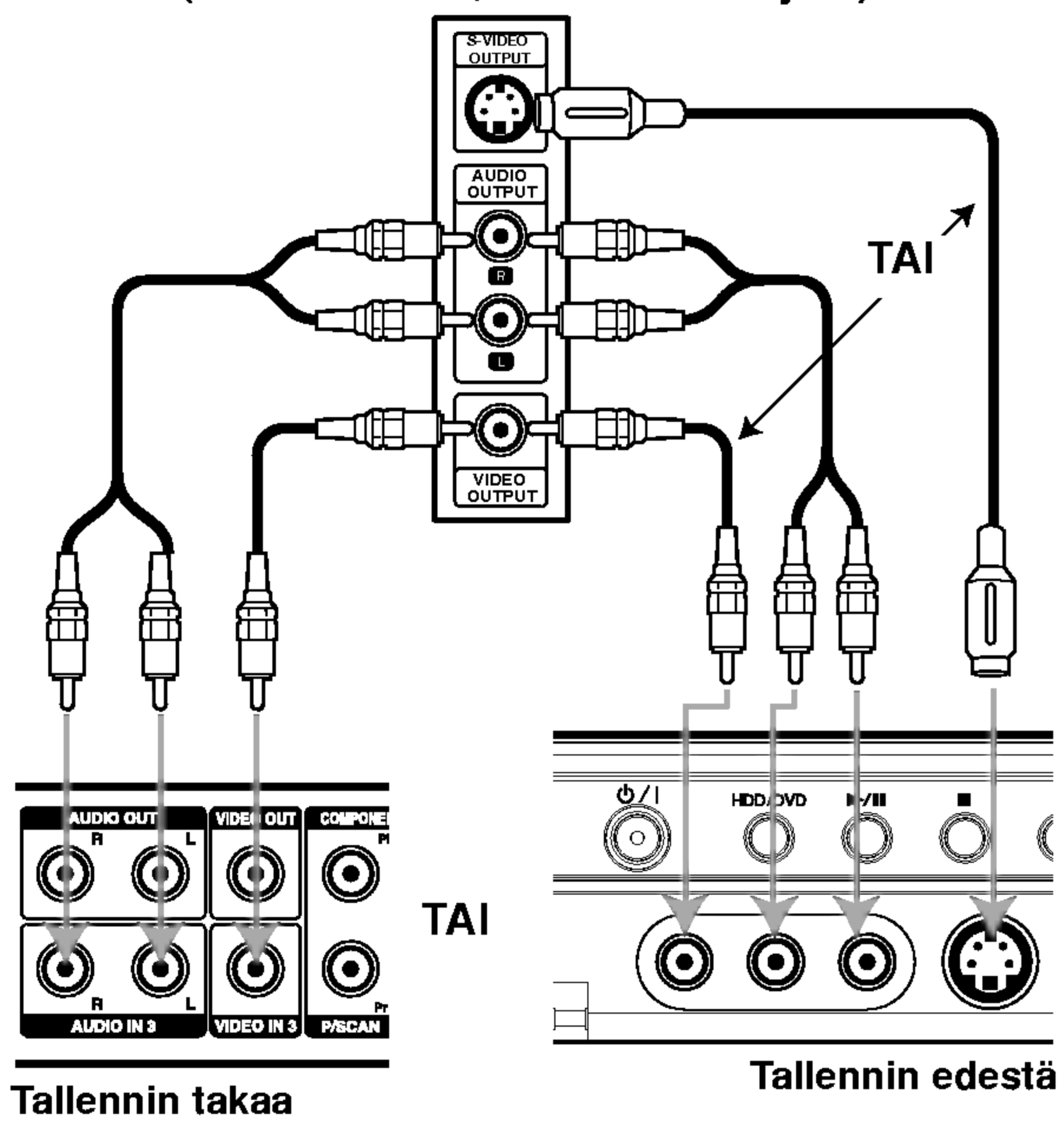
Liitinpaneeli lisälaitteille (videonauhuri, videokamera jne.)
